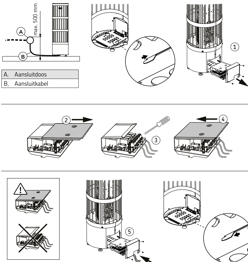
Figuur 5a. Elektrische aansluitingen
