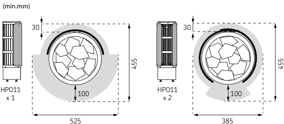
Figura 2. Distanze minime di sicurezza con guaina/e di protezione HP011 (accessorio opzionale)
