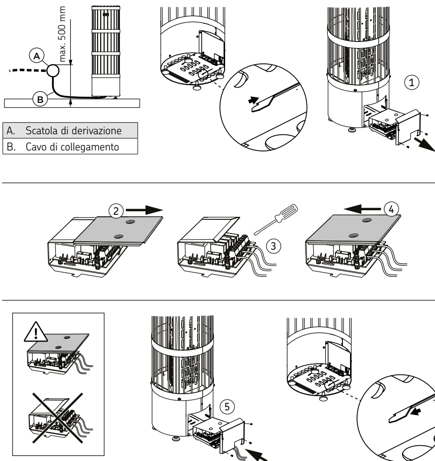
Figura 5a. Collegamenti elettrici
