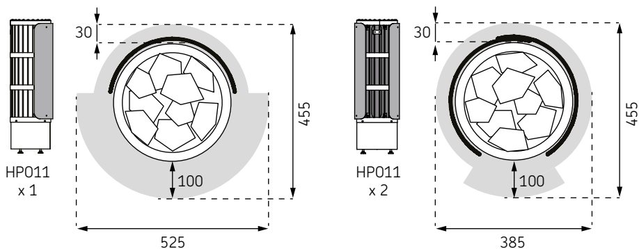
Kuva 2. Minimisuojaetäisyydet suojaseiniin (HP011) kanssa (Valinnainen lisävaruste).
