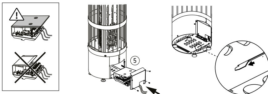
5.a attēls. Elektroapgādes pieslēgumi
