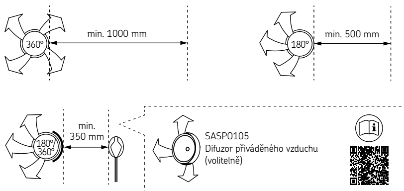
Obrázek 4 Minimální vzdálenost od větracího otvoru přívodu vzduchu k teplotnímu senzor
