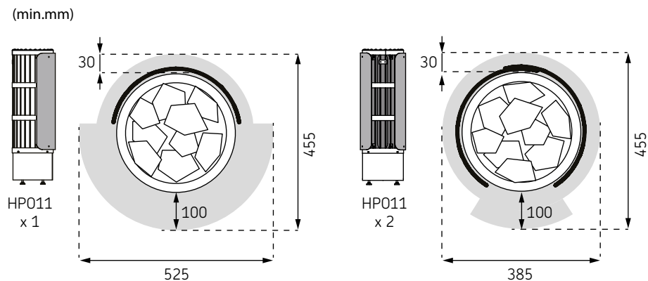
Рисунок 2. Минимальные безопасные расстояния с защитным чехлом (чехлами) HP011 (дополнительные аксессуары)
