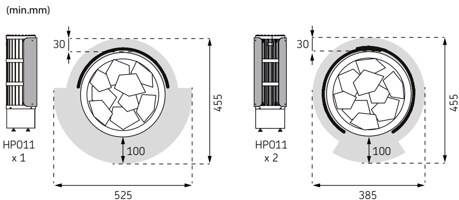
Joonis 2. Minimaalne ohutuskaugus koos kaitsekattega/-katetega HP011 (lisavarustus)
