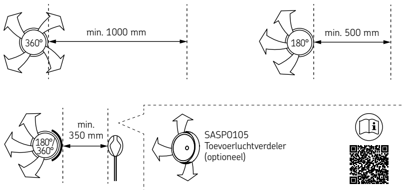
Figuur 4. Minimale afstand van de luchttoevoerklep tot de temperatuursensor
