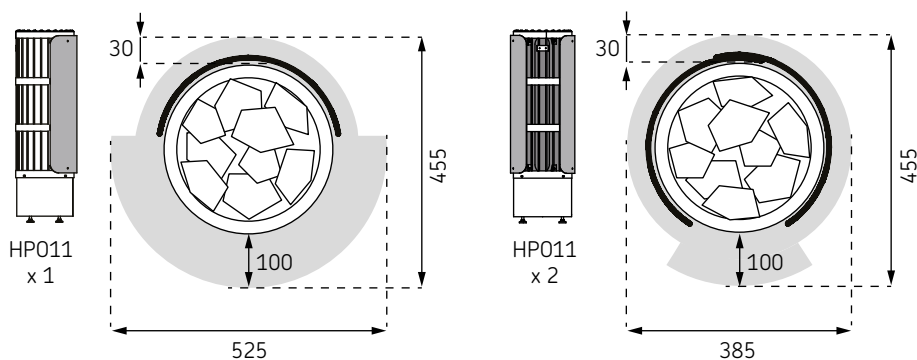
Abbildung 2. Mindestsicherheitsabstände mit Schutzmantel HP011 (optionales Zubehör)
