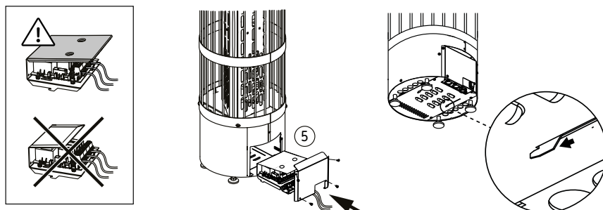
Slika 5a. Električni priključki
