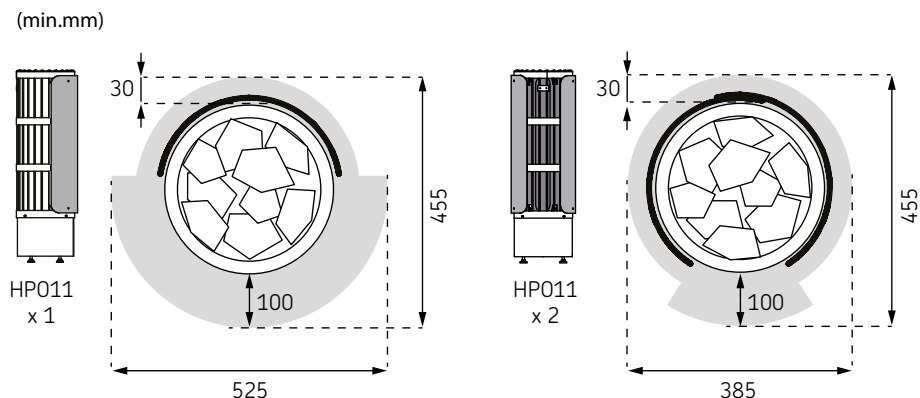
2. attēls. Minimālie drošie attālumi ar aizsargapvalku(-iem) HP011 (papildu piederumi pēc izvēles)
