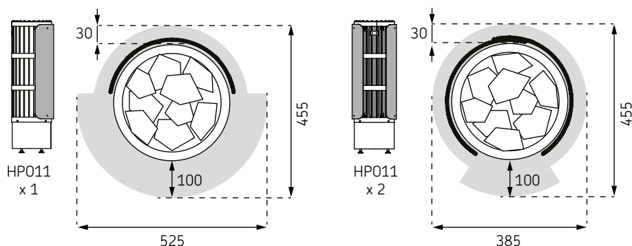
Figuur 2. Minimale veiligheidsafstanden met beschermmantel(s) HP011 (optioneel accessoire)
